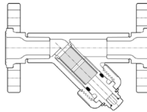
FLANGE
